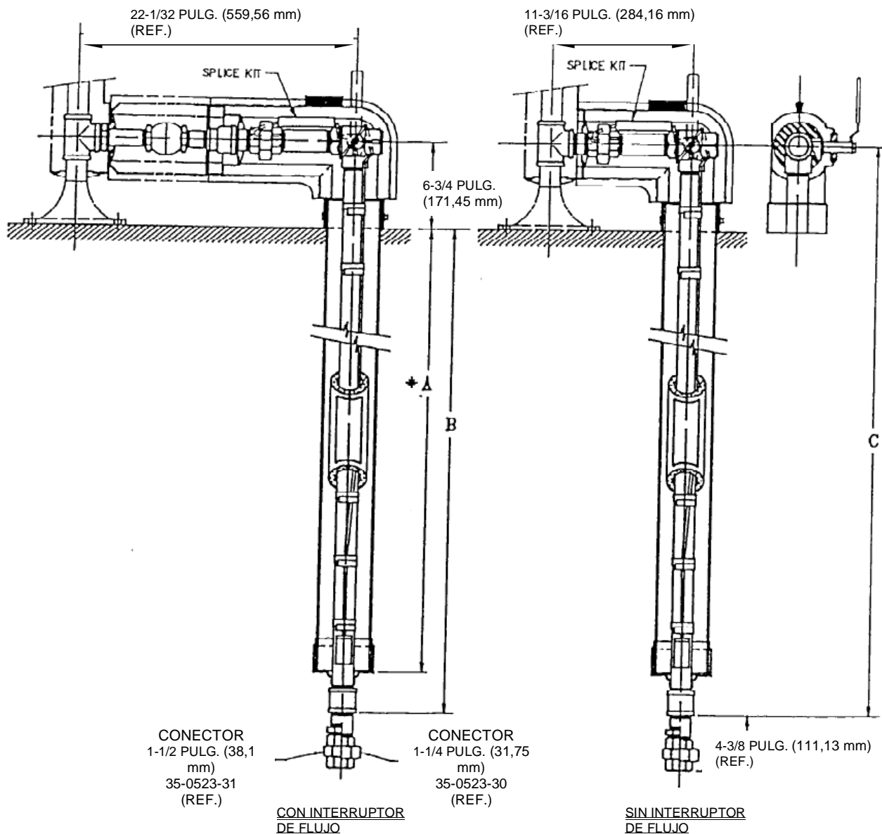
Figura 5. EXTENSION SUBTERRANEA (CON Y SIN INTERRUPTOR DE FLUJO)
