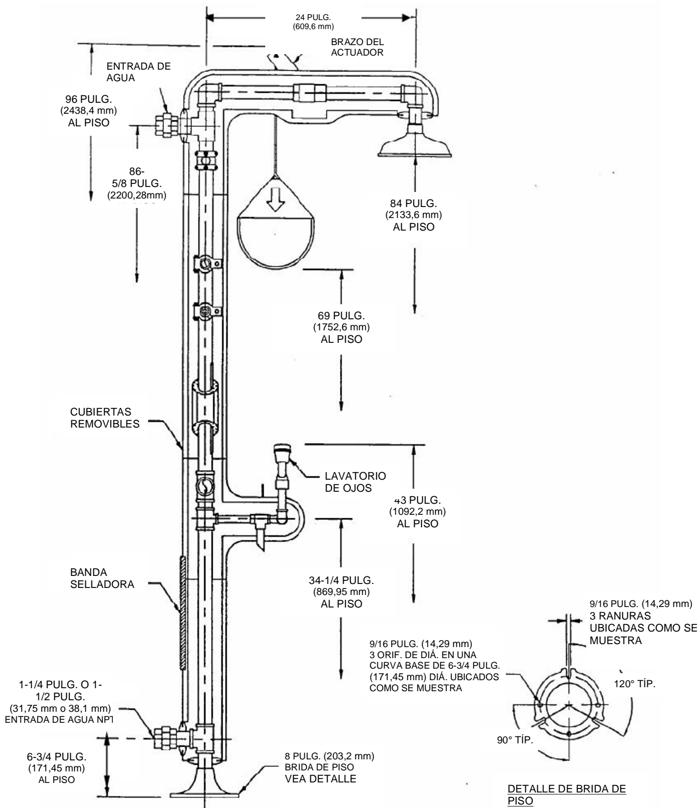
Figura 1A. DIMENSIONAL, DUCHA DE EMERGENCIA
