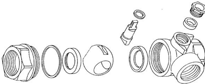
Figura 3C. CONJUNTO VÁLVULA DE BOLA LAVATORIO DE OJOS
